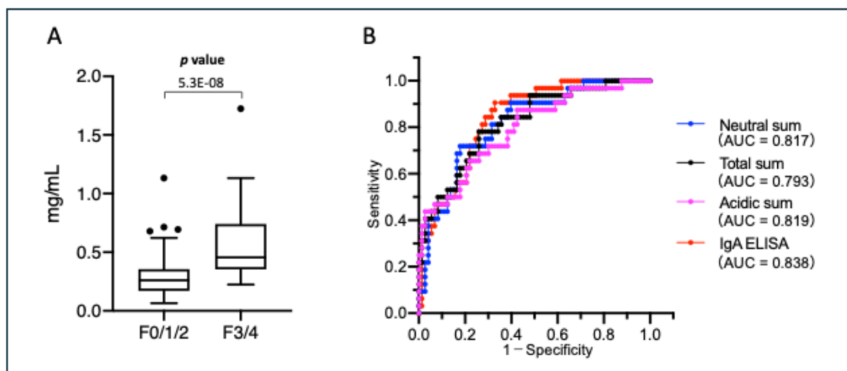
図 2 (A) サンドイッチ ELISA によるバイセクト N 型糖鎖が結合した IgA タンパク質の測定。高度線維化群 (F3/4) で有意に増加。(B) バイセクト N 型糖鎖群の様々な合算値 (Neutral sum: 中性糖鎖のみで構成されるバイセクト N 型糖鎖の合計、Acidic sum: シアル酸バイセクト N 型糖鎖の合計、Total sum: バイセクト N 型糖鎖の合計) および サンドイッチ ELISA の ROC 解析。
